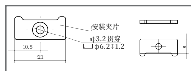
LP-AJ-2 安装夹片
